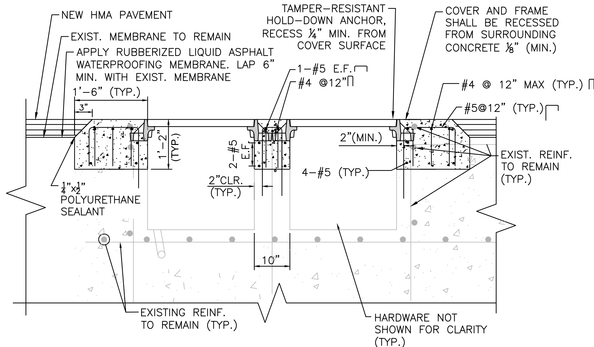
SECTION C SCALE: 3/4"=1'-0"
