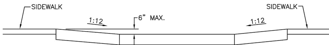
ELEVATION
